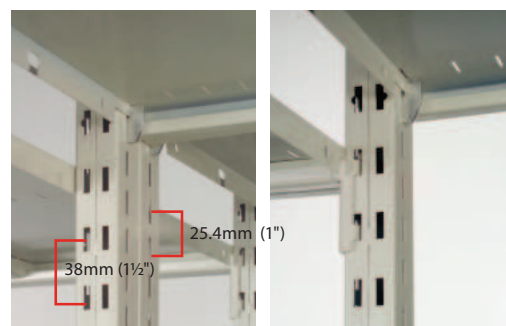
Deux technologies dans un cadre à montant unique. Illustré sans panneau de fermeture ni séparateur d'extrémité optionnels Brevet no° 6,814,245
