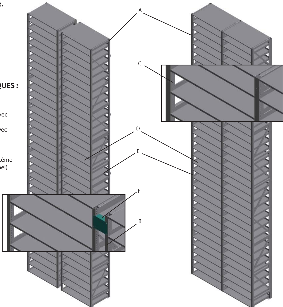
Configuration initiale-allonge
